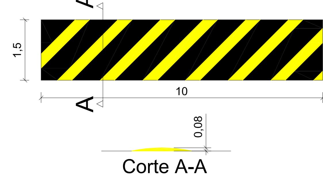
5 SINALIZAÇÃO HORIZONTAL - LOMBADA
