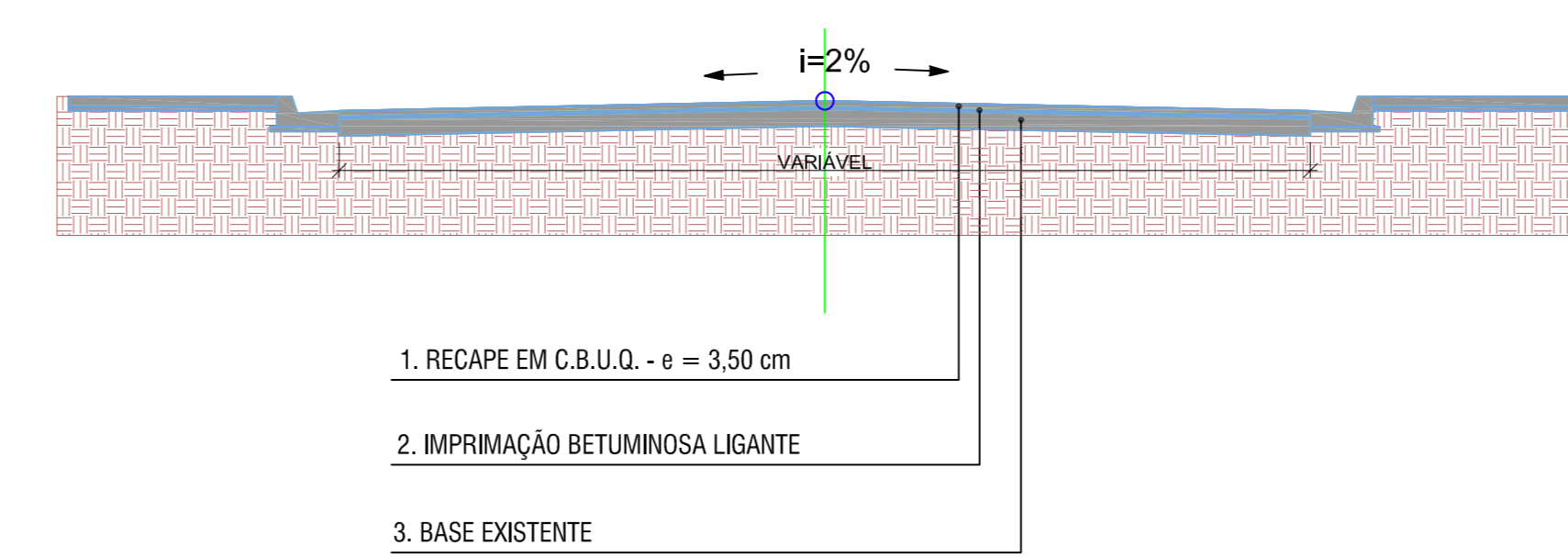
3 SEÇÃO TÍPICA DO PAVIMENTO ESCALA: 1:50
