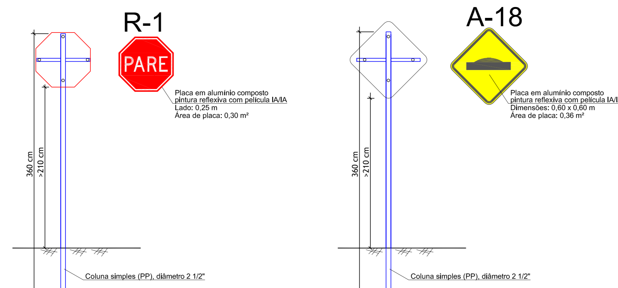
6 SINALIZAÇÃO VERTICAL
