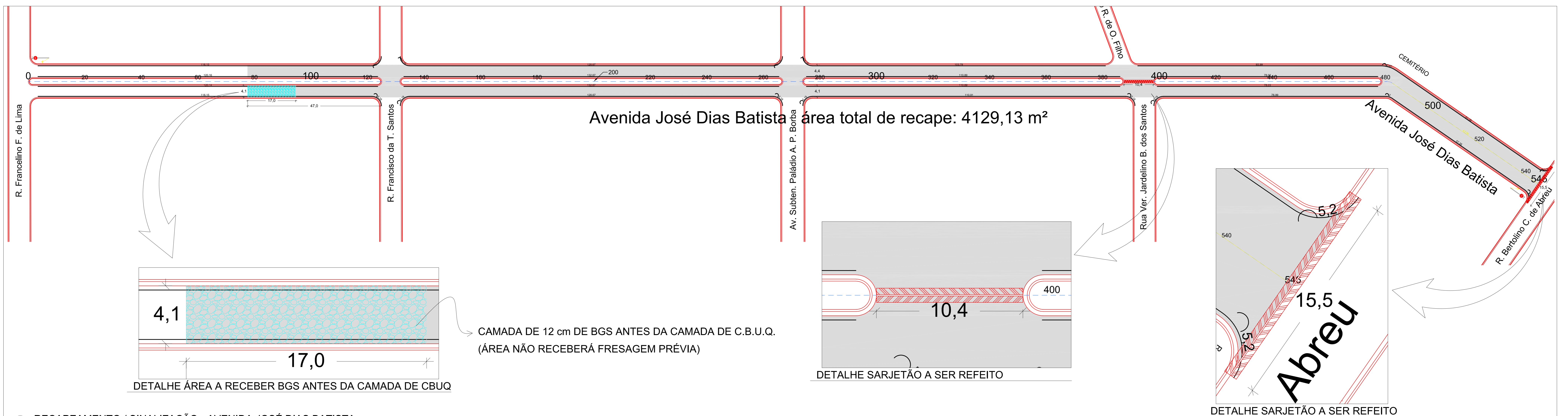
1 RECAPEAMENTO / SINALIZAÇÃO - AVENIDA JOSÉ DIAS BATISTA ESCALA: 1:500
