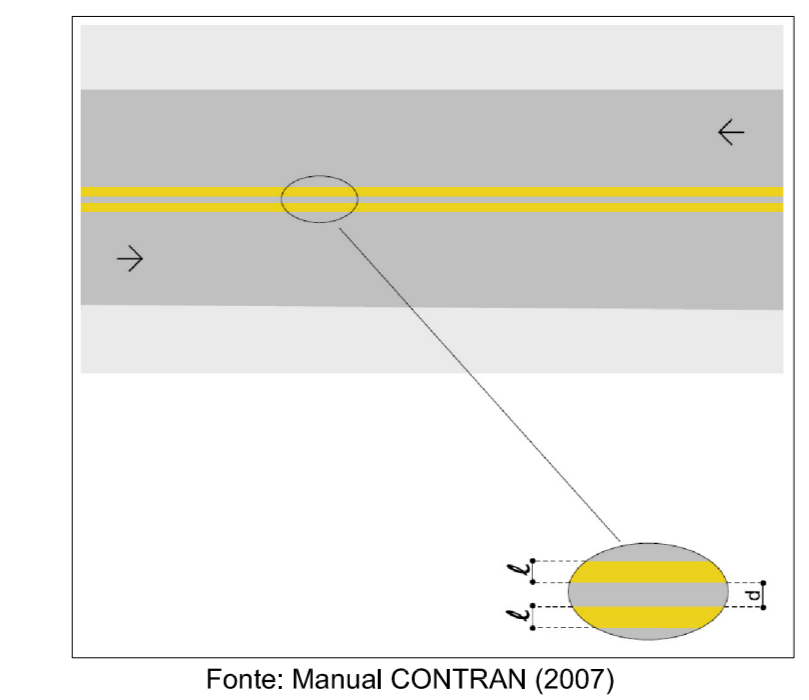
LINHA DUPLA CONTÍNUA (LFO-3)
