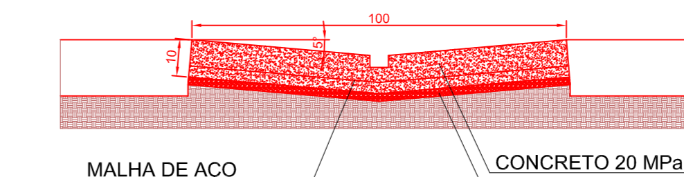
7 DETALHE SARJETÃO
