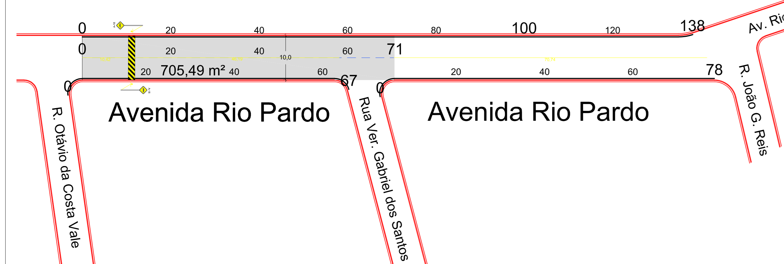
2 RECAPEAMENTO / SINALIZAÇÃO - AVENIDA RIO PARDO ESCALA: 1:500
